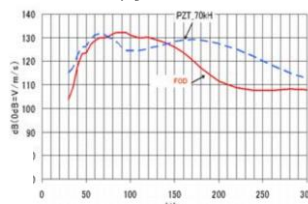
周波数特性表
